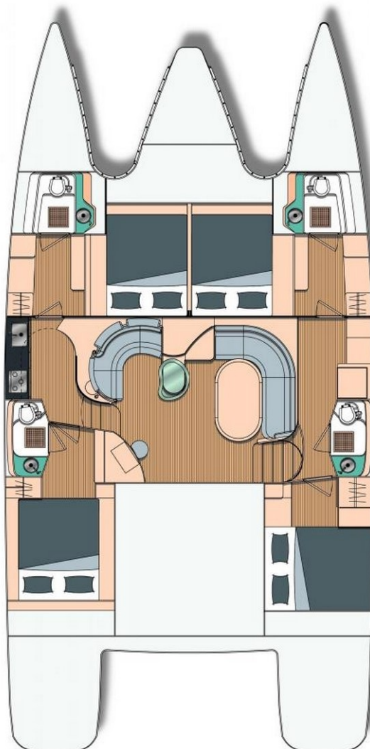
Plan d'aménagement standard - Version 4 cabines
